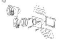
Válvula de láminas 125
