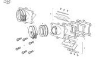
Válvula de láminas 200-250-300
