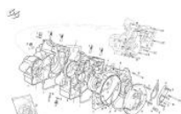
Carter de motor 200-250-300
