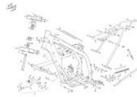
Chasis
