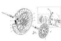
Rueda delantera SM
