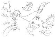
Carrocería MC
