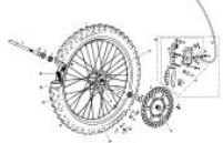
Rueda delantera MC
