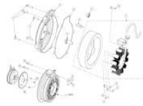
Generador
