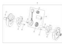
Cigüeñal
