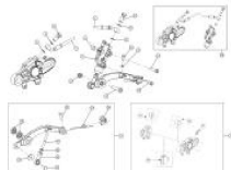
Freno trasero
