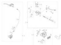
Freno delantero
