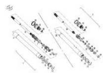
Horquilla delantera
