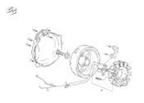
Generador 125-200
