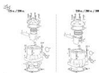
Cilindro
