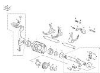
Arbol selector cambio
