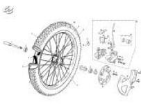
Rueda delantera
