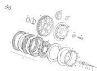
Embrague
