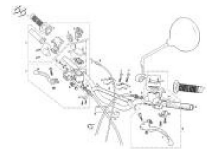
Manillar - mandos
