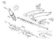
Basculante
