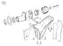
Admisión
