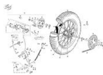
Rueda trasera
