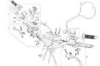
Manillar - mandos
