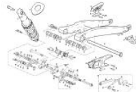
Basculante
