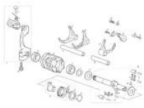
Arbol selector cambio
