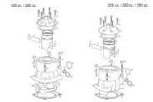
Cilindro - Culata
