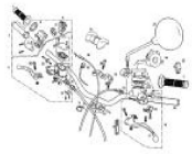
Manillar - Mandos
