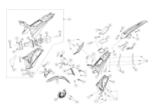
Montaje plásticos
